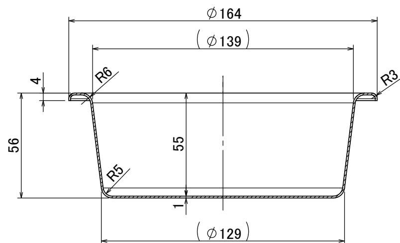
断面図 A-A
