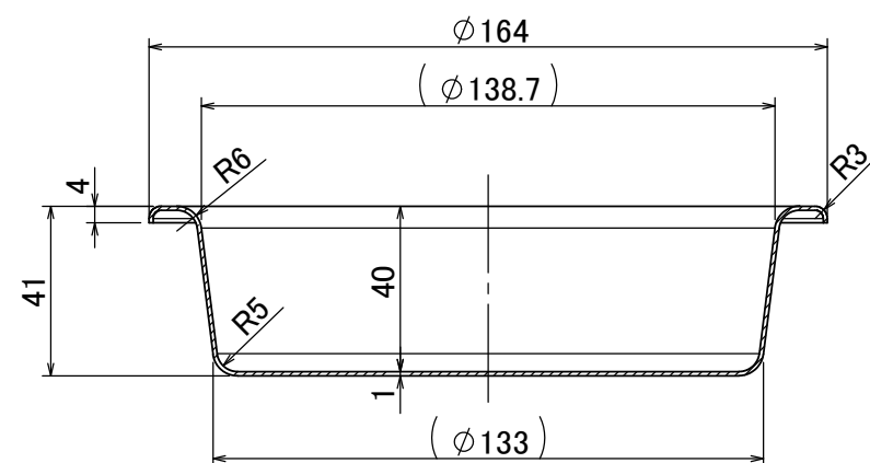
断面図 A-A
