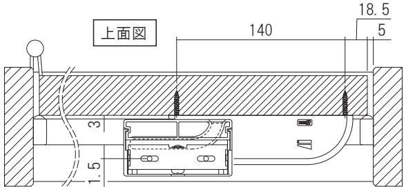
受けスプール (R勝手)
