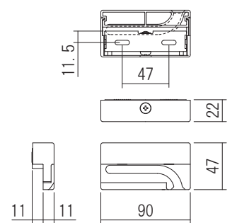
受けスプール (R勝手)
