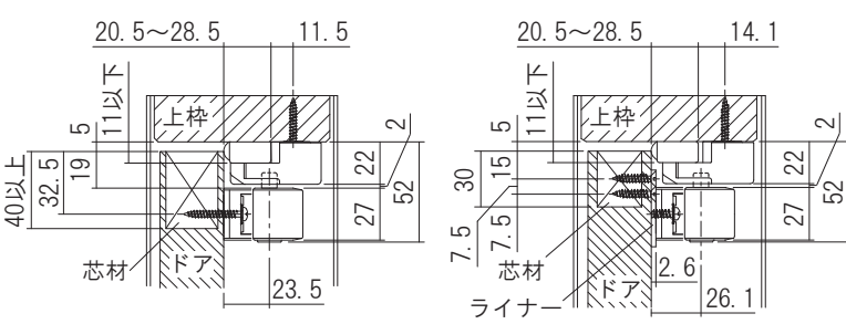
ドア取付け用ライナー無し
