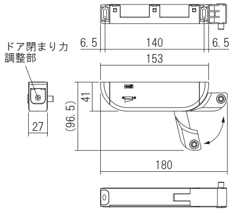
本体 (L勝手)
