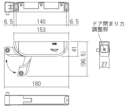
本体 (R勝手)
