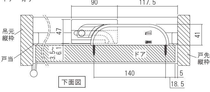
取付参考図 (図はR勝手を表す)
