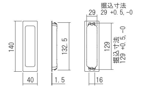
上図は角型の場合、丸型も同掘り込み
