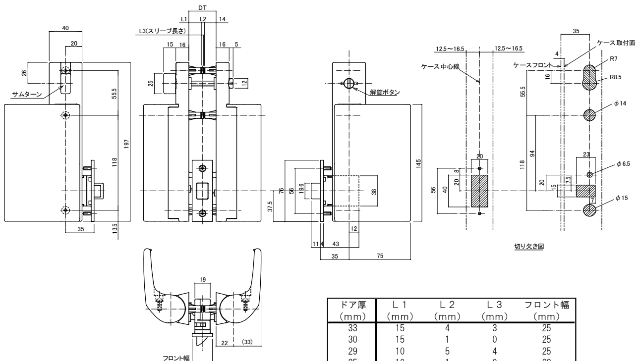
门厚和各个部位尺寸
