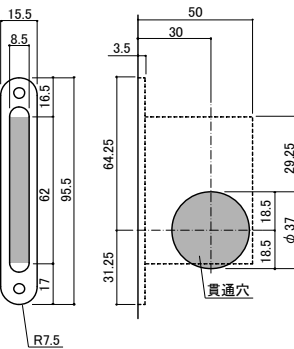
锁盒用门框加工图
