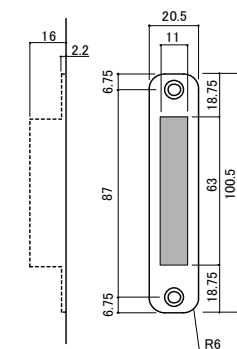
锁座用门框加工图
