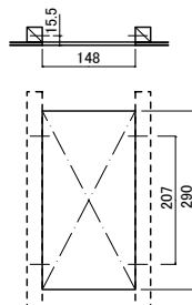
掘り込み加工図
