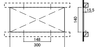
掘り込み加工図
