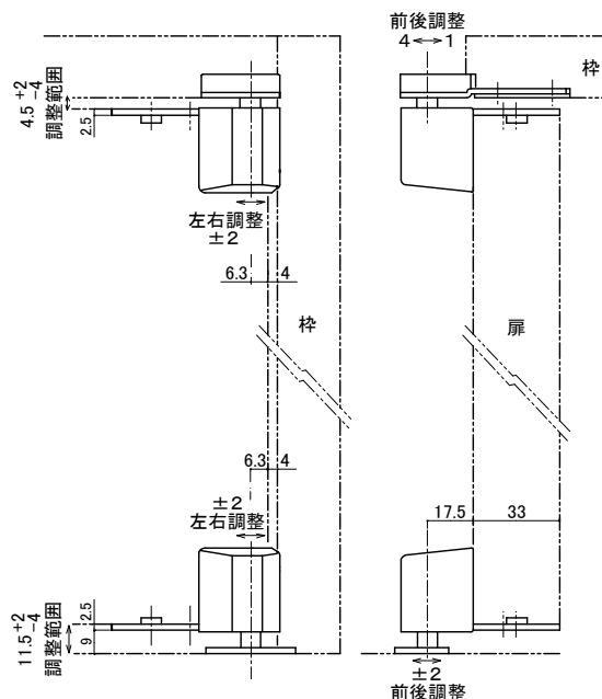
取付参考図
