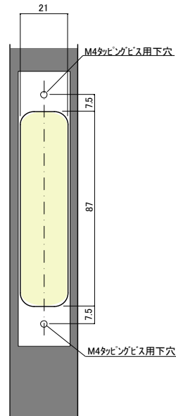
切り欠き図
