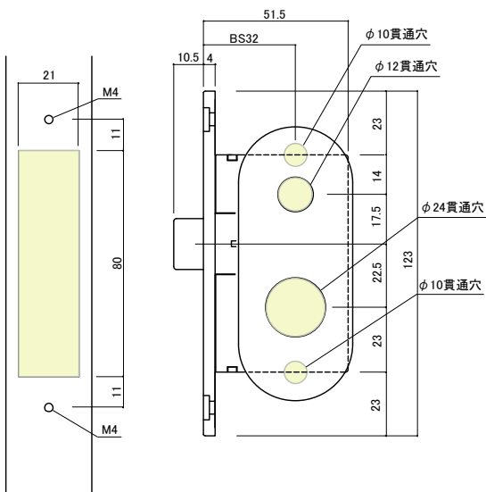
アルミ框ドアの場合
