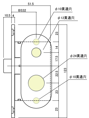
小判座(D・J型)間仕切り・表示錠
