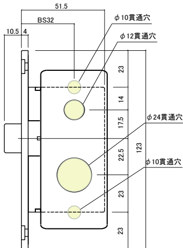
アルミ框ドアの場合
