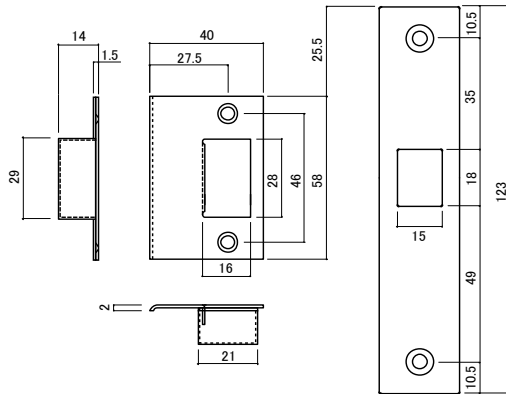
角座(F型)間仕切り・表示錠
