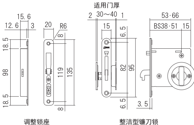
调整锁座
