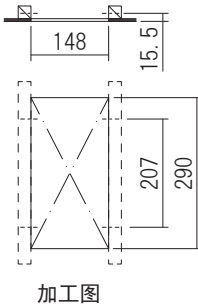
加工图
