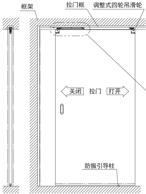
安装参考图
