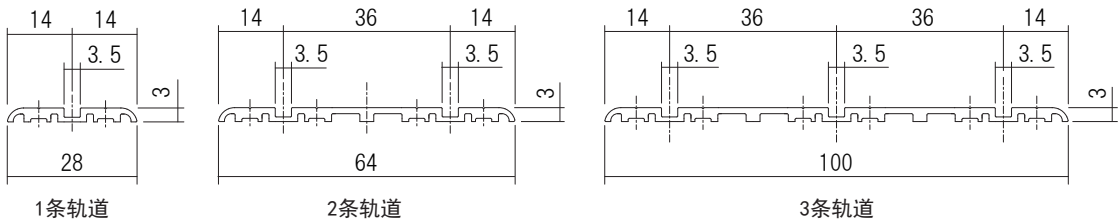
1条轨道
