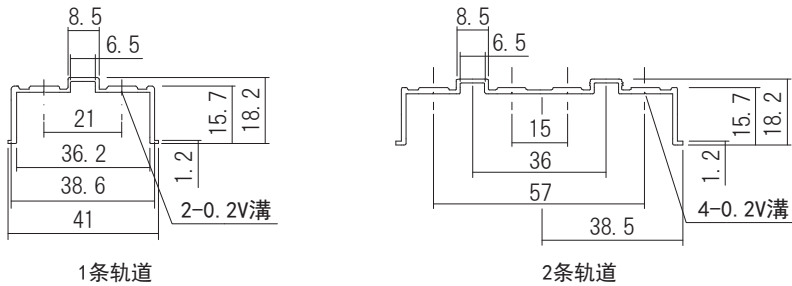
1条轨道
