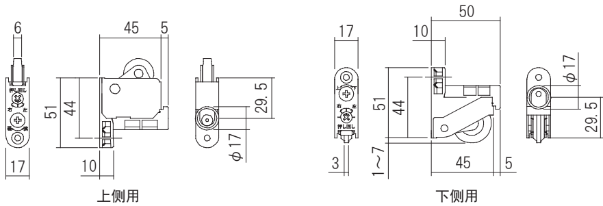
上侧用
