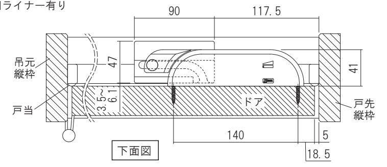
取付参考図 (図はR勝手を表す)
