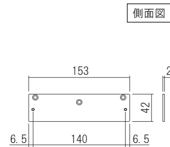
ドア取付け用ライナー
