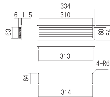
切り欠き図
