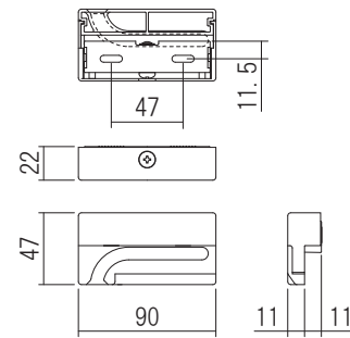
受けスプール (L勝手)
