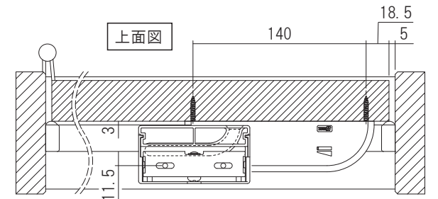
受けスプール (R勝手)
