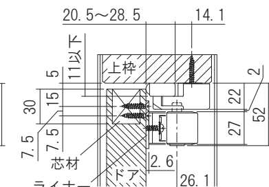
ドア取付け用ライナー有り
