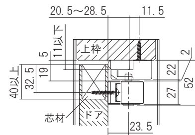
ドア取付け用ライナー無し
