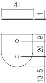
パッキン
