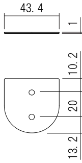
パッキン
