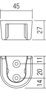
ブラケット
