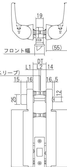
室内側 (左勝手)
