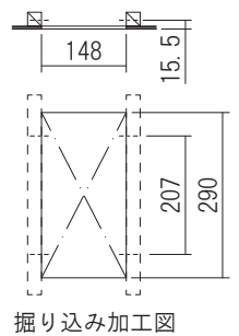
掘り込み加工図
