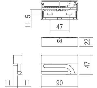
受けスプール (R勝手)
