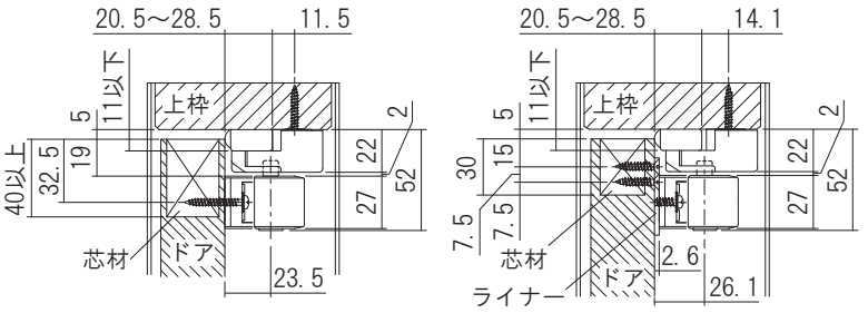
ドア取付け用ライナー無し
