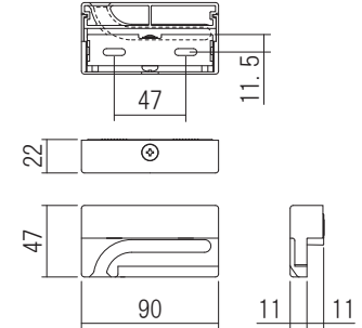
受けスプール (L勝手)
