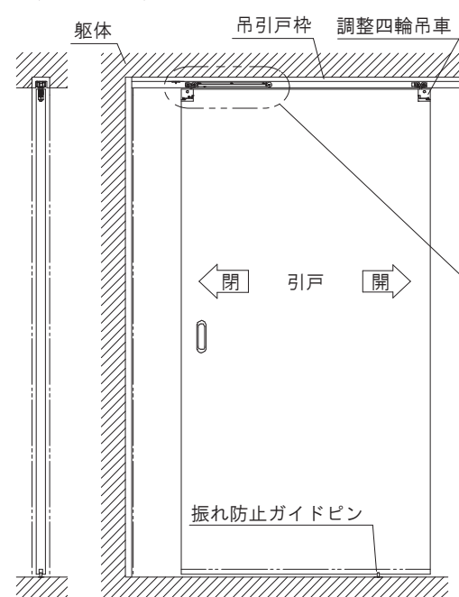
取付参考図
