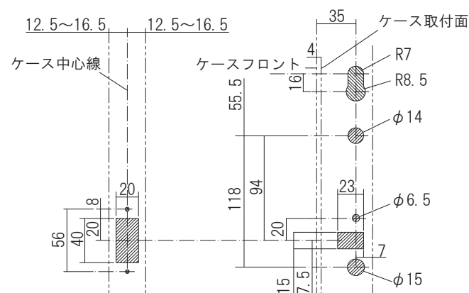
切り欠き図
