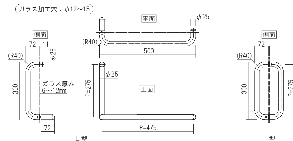
L型
