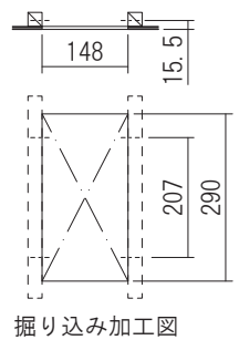
掘り込み加工図
