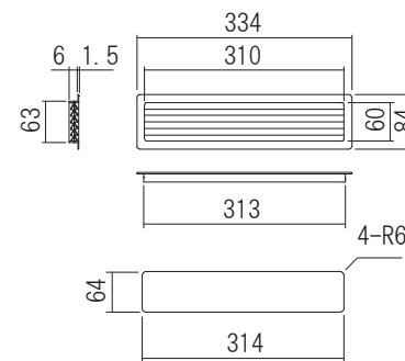
切り欠き図
