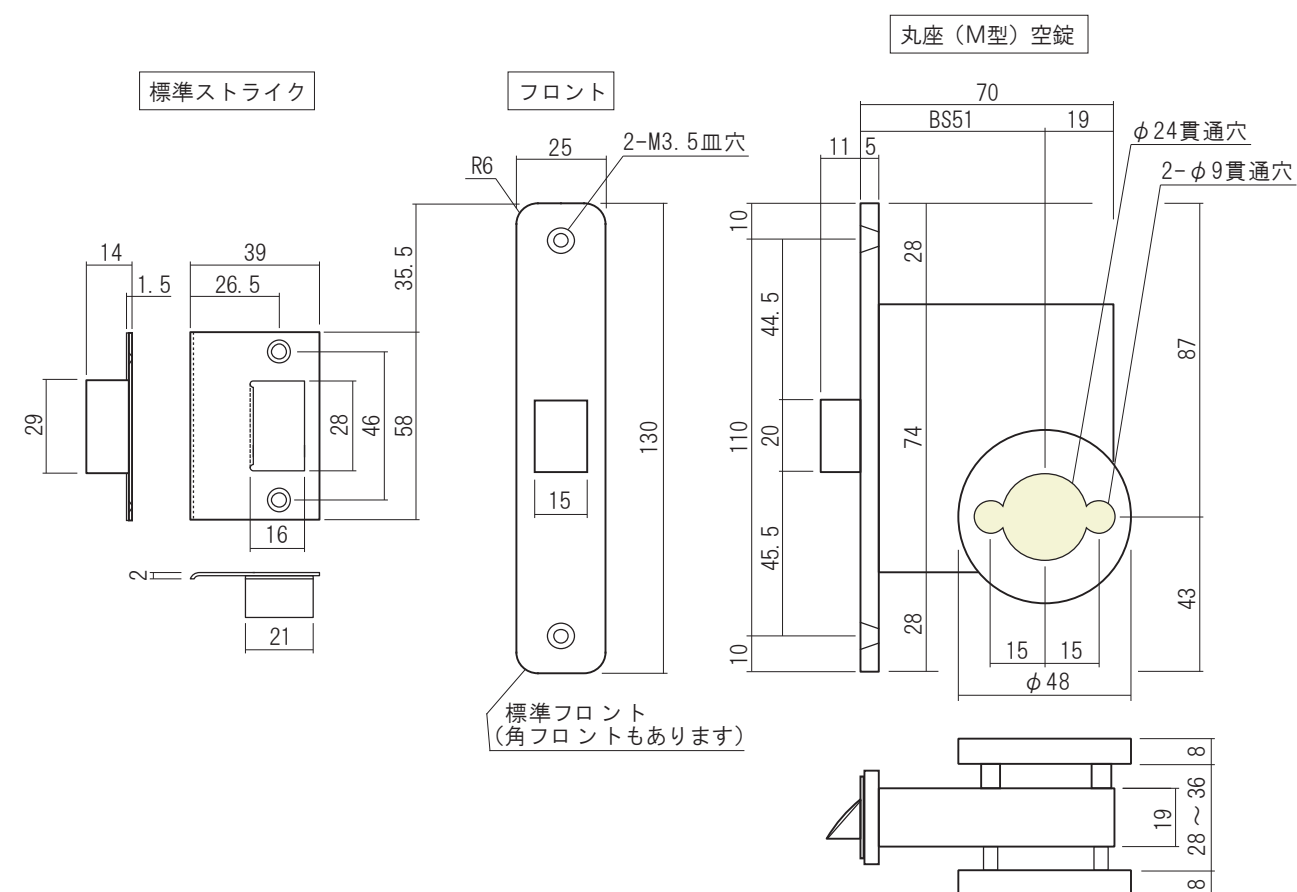
FRケース切欠外形図 ■標準扉厚 2 8 ~ 3 6 mm
