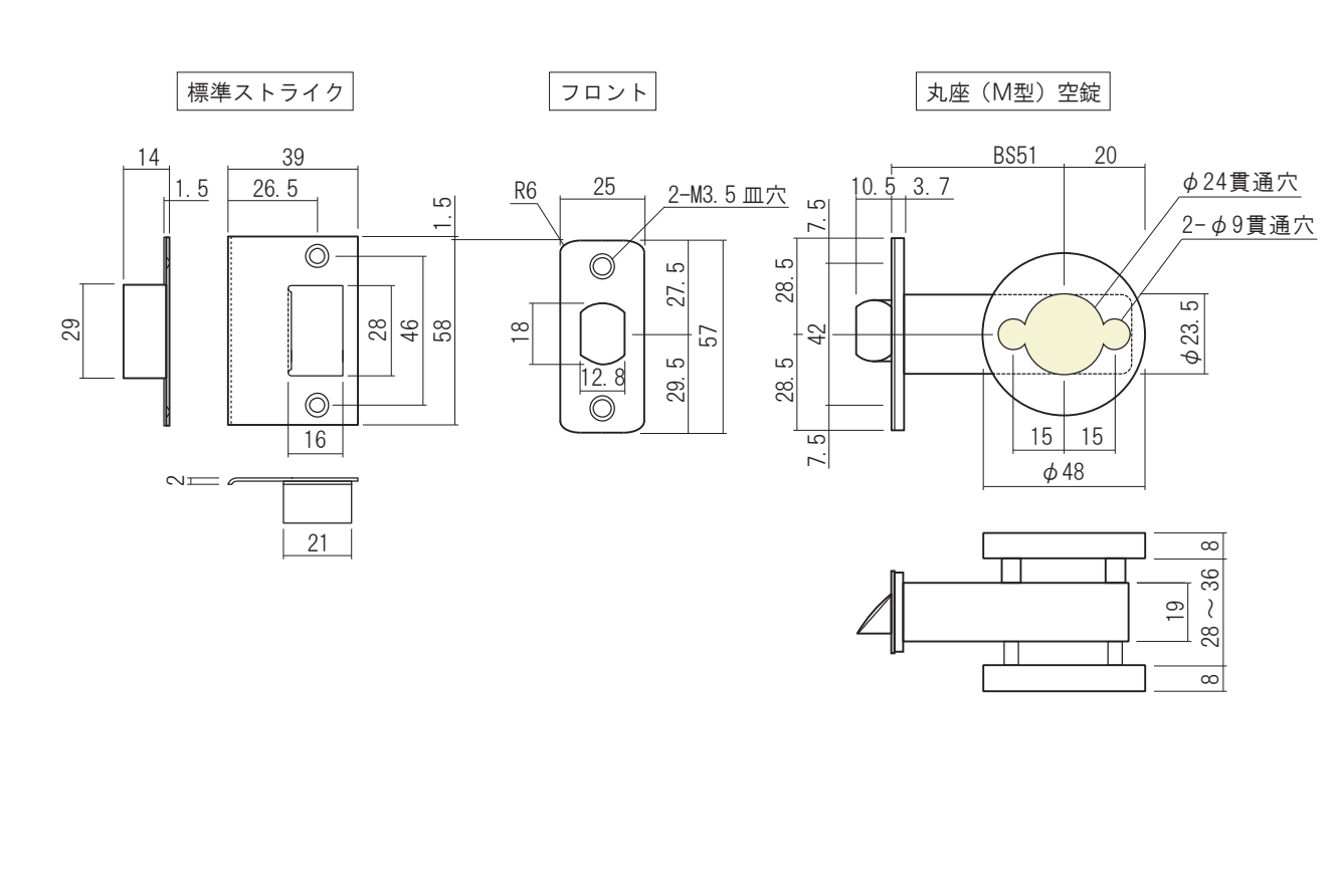
FTケース切欠外形図 ■標準扉厚 2 8 ~ 3 6 mm
