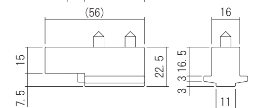
レール内ストッパー
