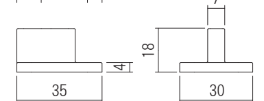
フロアーガイド
