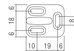
レール内ストッパー
