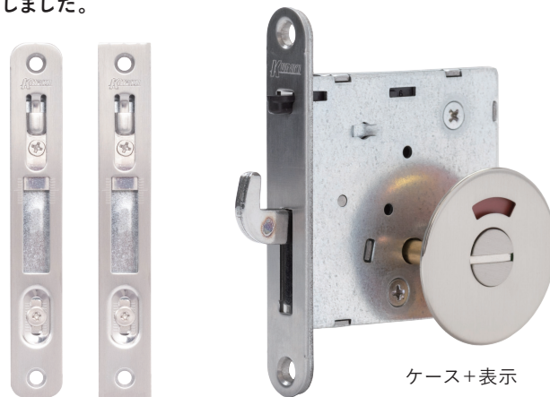
丸型 角型 調整ストライク (下鎌錠)
