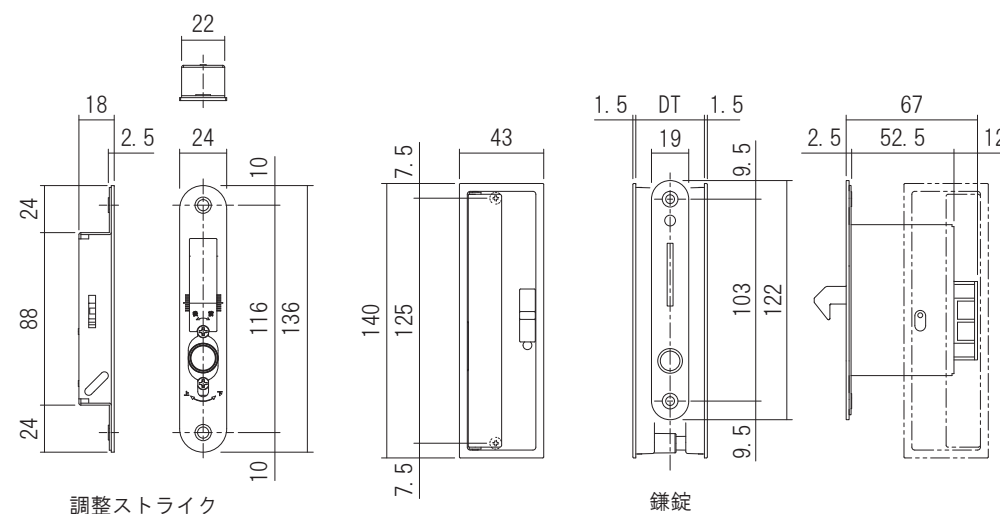
調整ストライク
