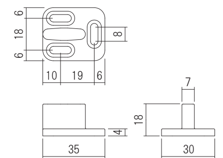
フロアーガイド
