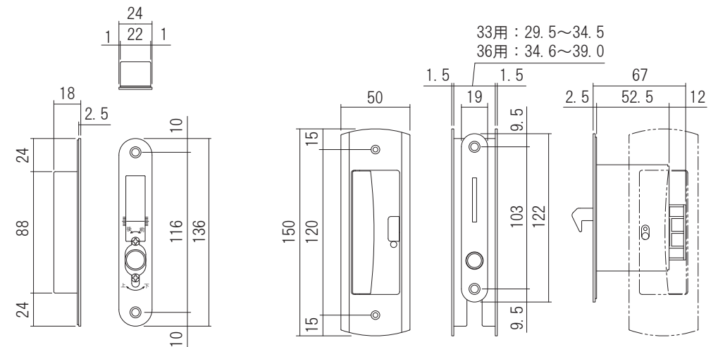
調整ストライク
