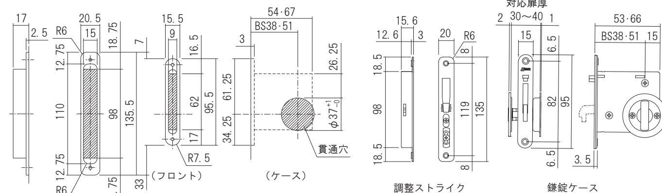
ストライク掘り込み図
