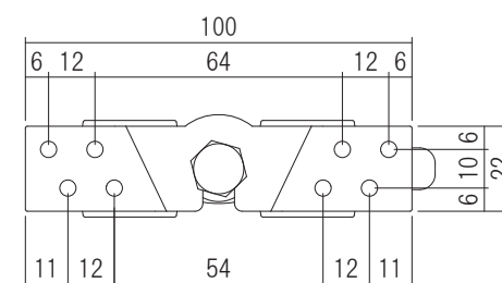
重量タイプ吊車
