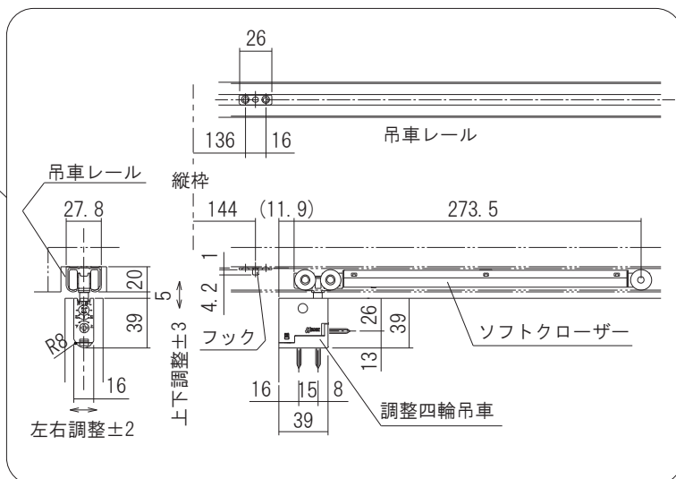
ソフトクローザー
