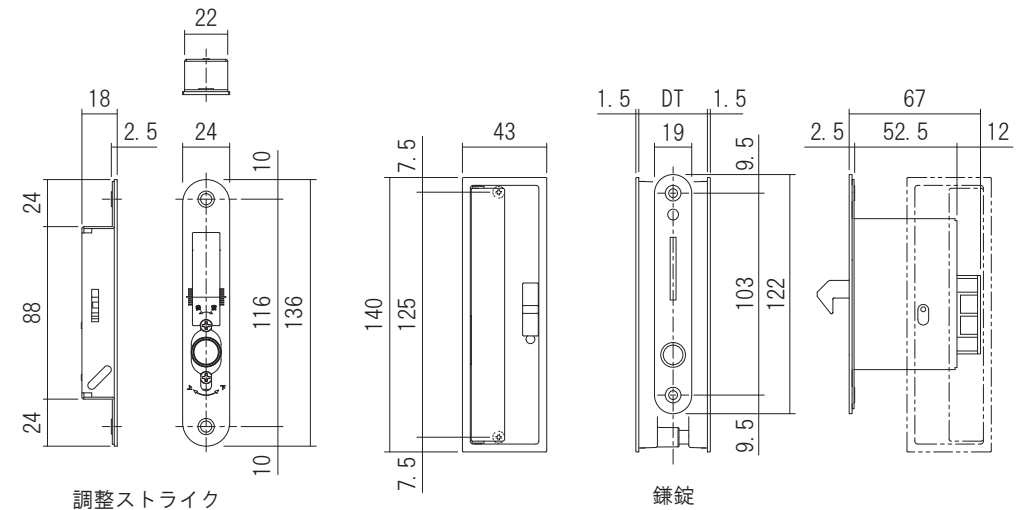
調整ストライク
