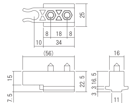
レール内ストッパー
