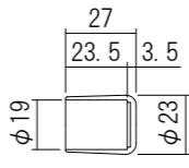
Cap
