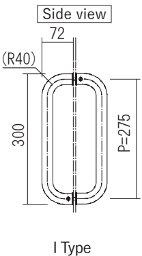
I Type
