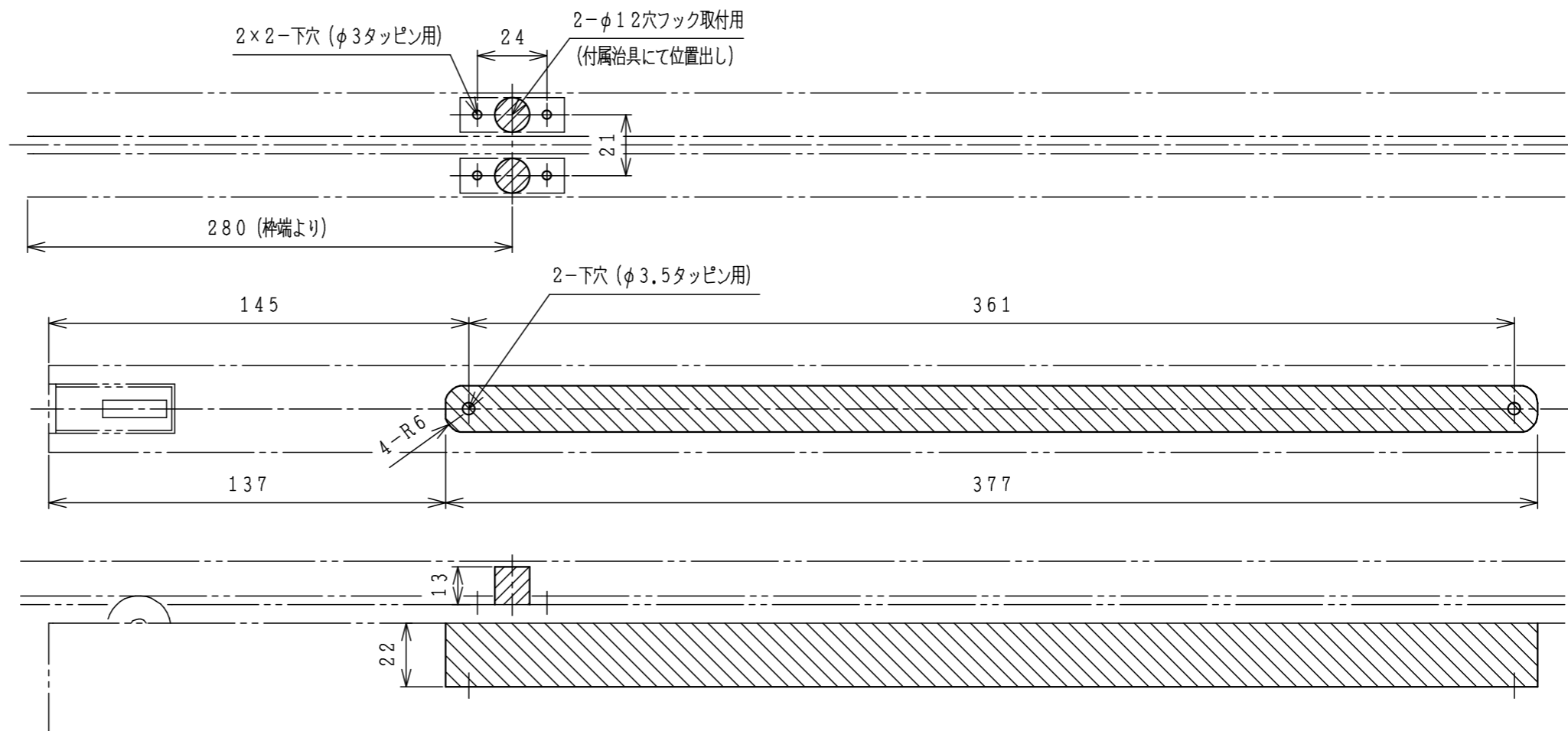
参考掘込図
