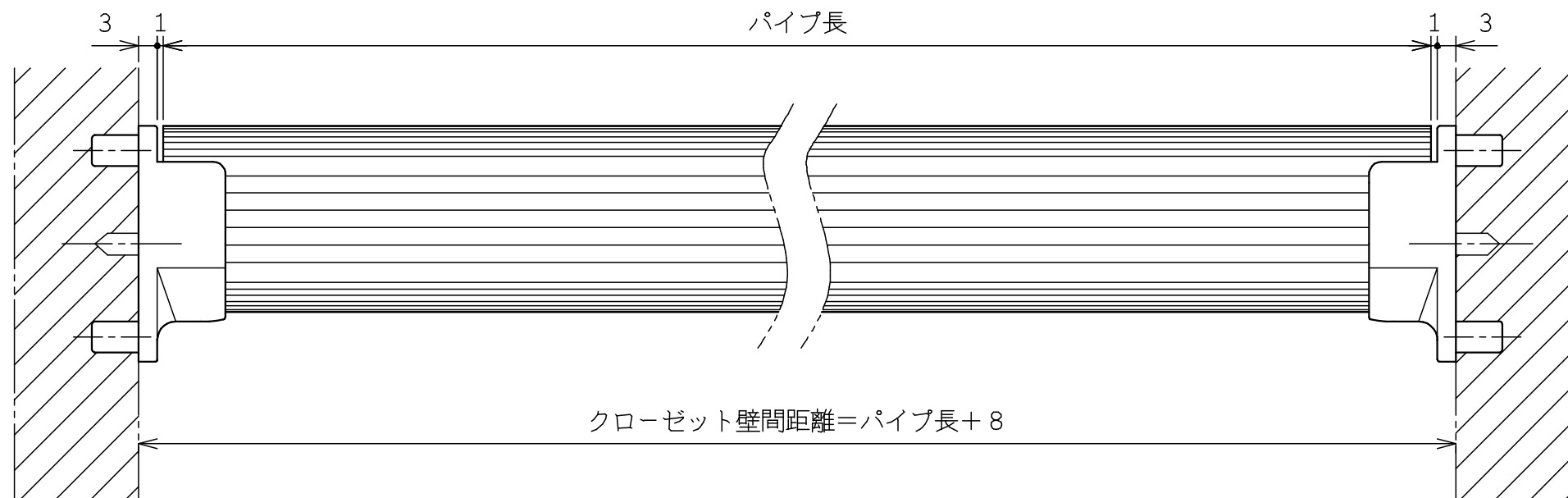
参考施工例
