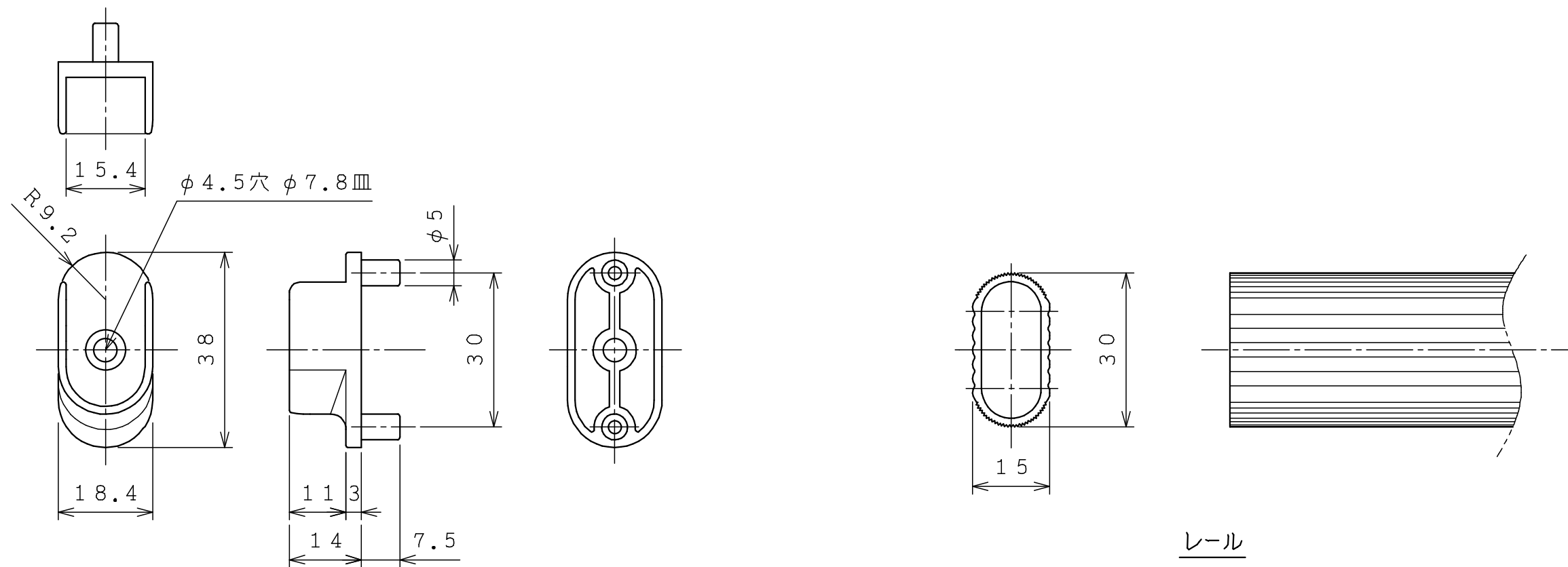
ブラケット
