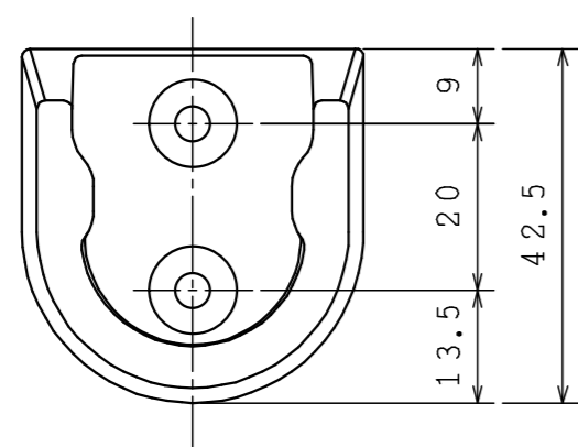
ブラケット
