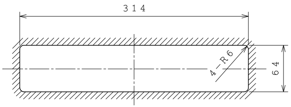
掘り込み参考図 (S=1:3)
