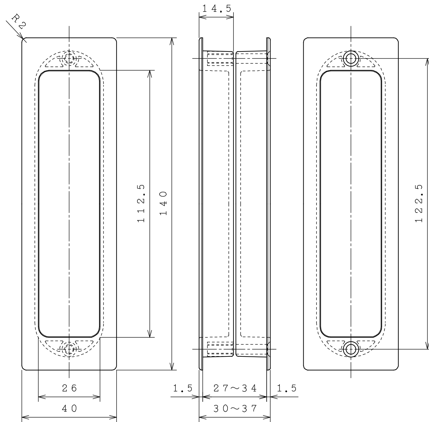
角型
