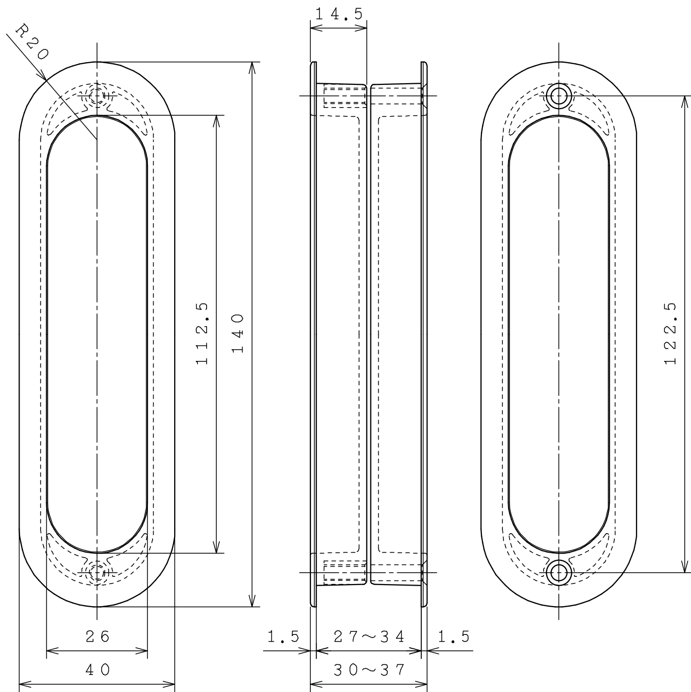
丸型
