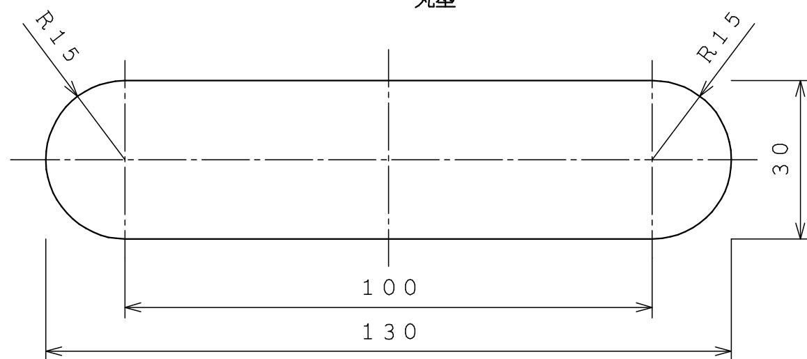
参考掘込図
