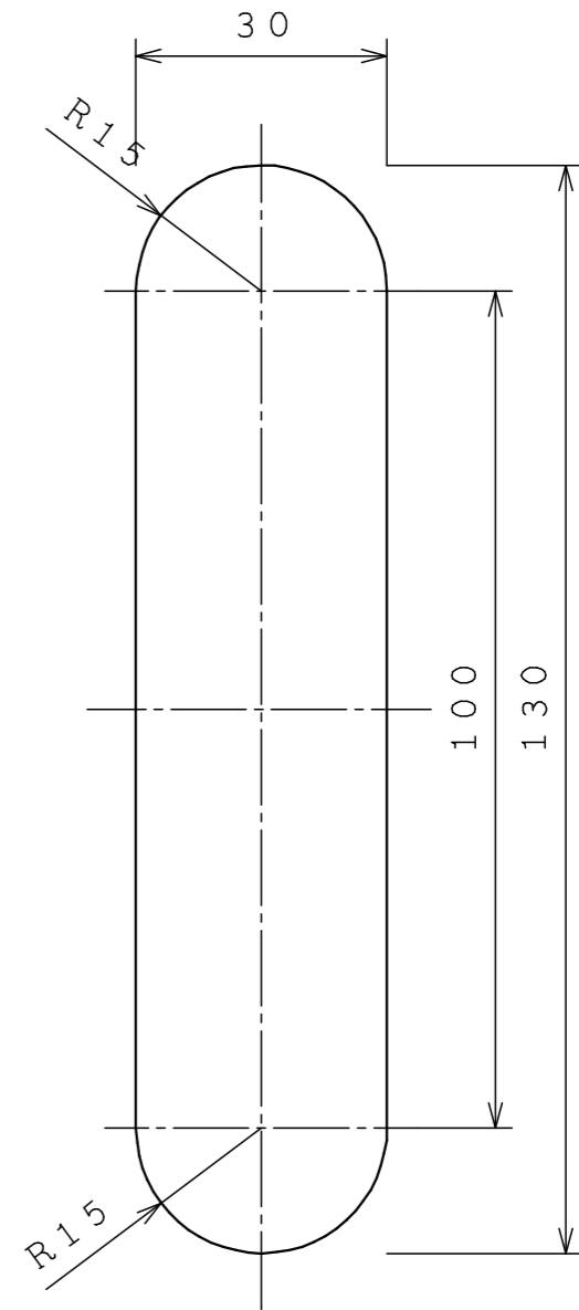
参考掘込図
