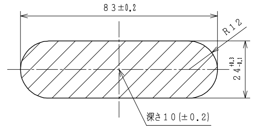
参考掘込図
