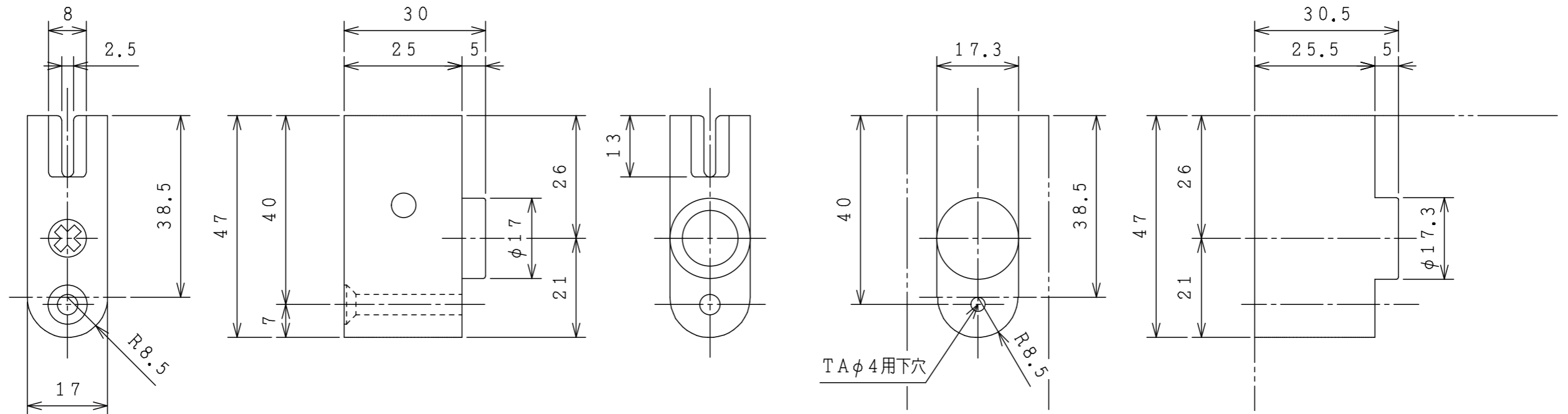
参考掘込図
