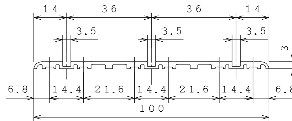
仕様：3本引き
