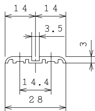
仕様：1本引き
