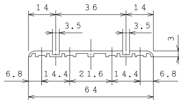
仕様：2本引き
