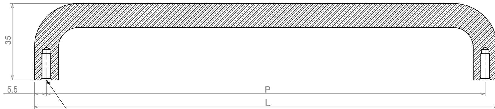
断面図 A-A
