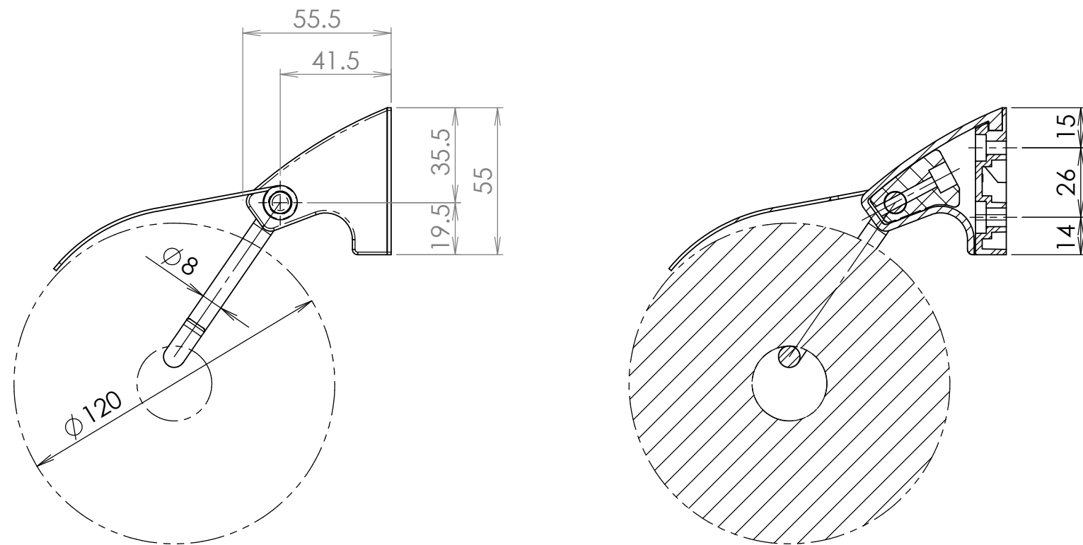
断面図 A-A
