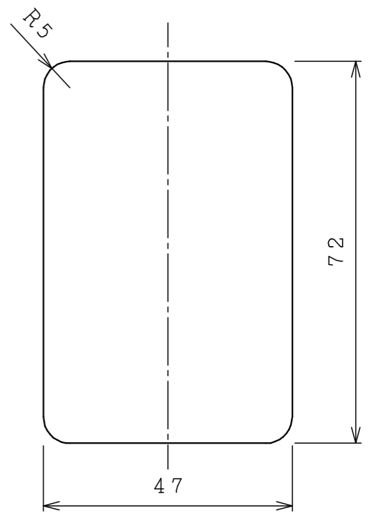
参考掘込図
