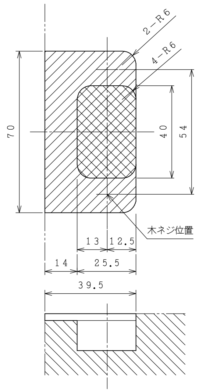
参考掘込図
