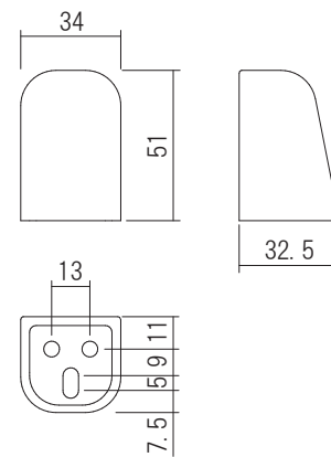
戸当り本体
