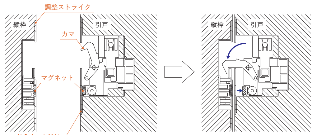
動作説明
