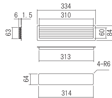
切り欠き図
