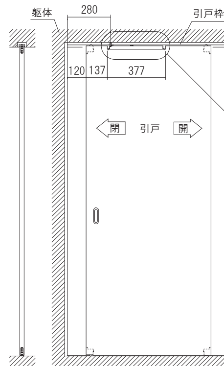
取付参考図
