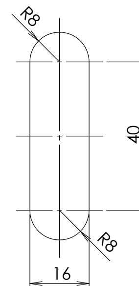
参考掘込図
