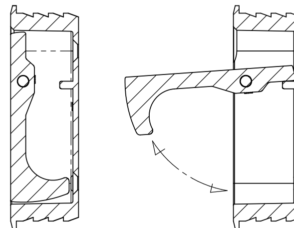
断面図 A-A
