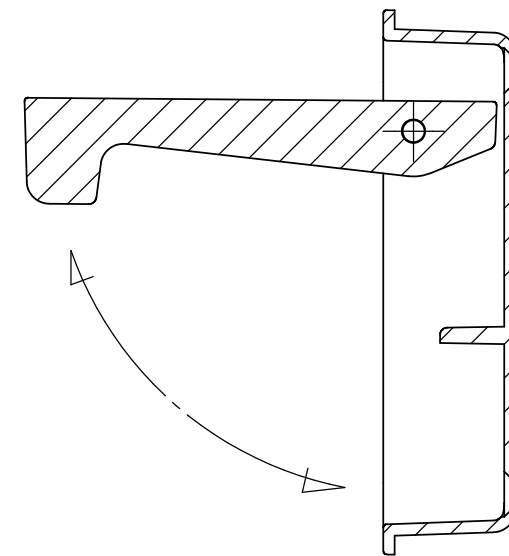
断面図 A-A
