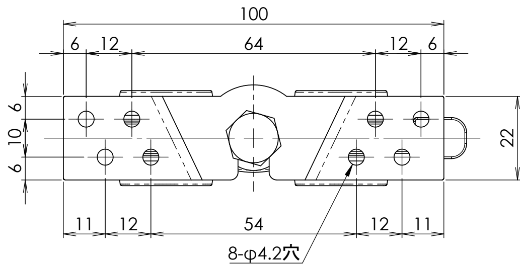
重量タイプ吊車
