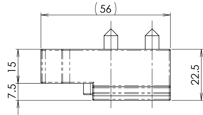
レール内ストッパー
